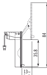
SPF/PCV Supporto pentola cottura a vapore per forno Oven steamer support
