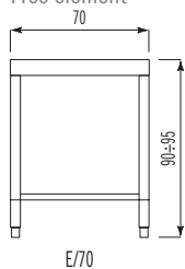
Elemento libero Free element
